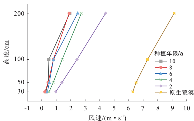
图 2 不同种植年限梭梭林不同高度的风速廓线的对比
