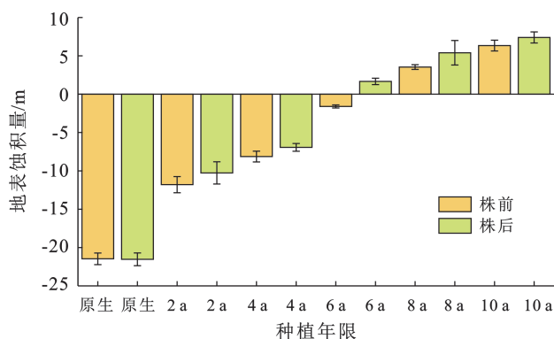
图 3 不同种植年限梭梭林地表蚀积量
