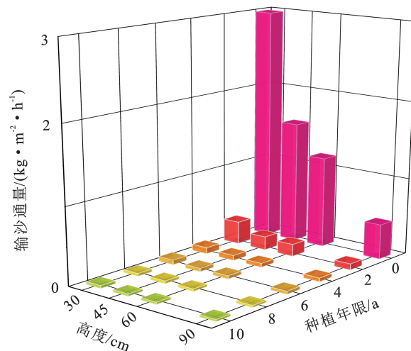
图 4 不同种植年限梭梭林不同高度输沙通量
