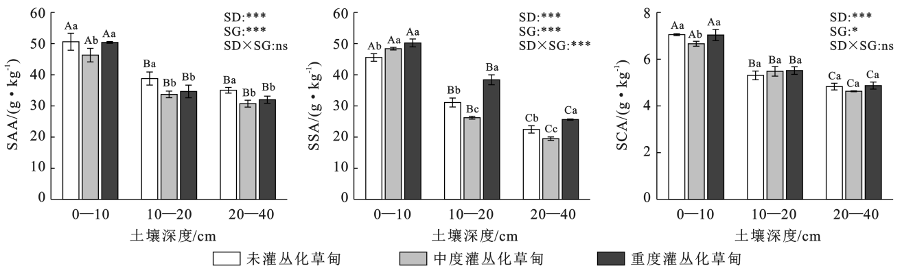
图 2 土壤酶活性分布特征
