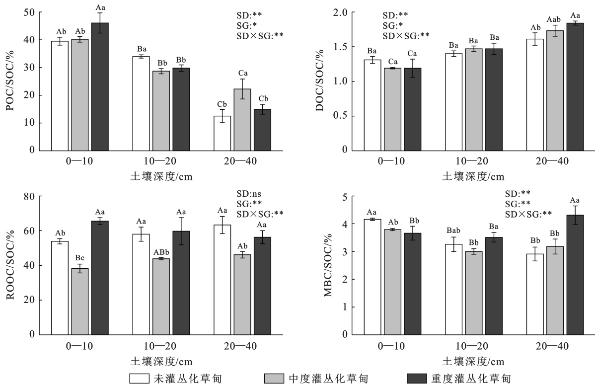
图 4 土壤有机碳活性组分占有有机碳比例分布特征
