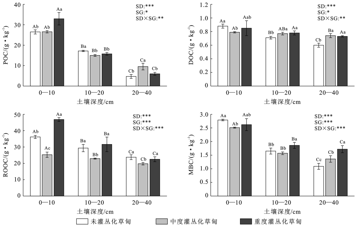
图 3 土壤有机碳活性组分分布特征
