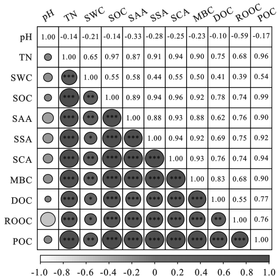
图 5 土壤各因子的相关性热图
