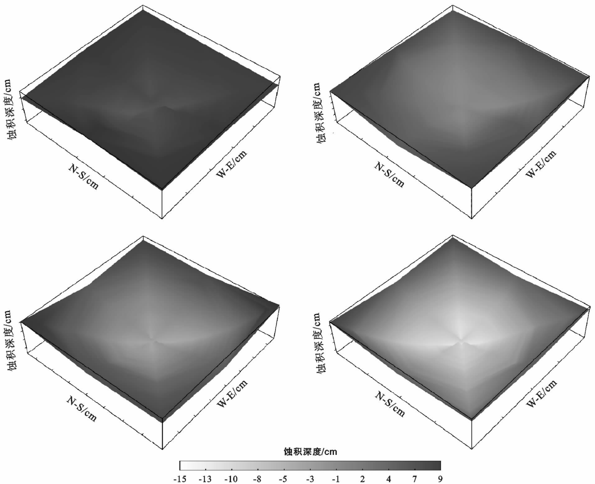
图 1 不同规格 PLA 沙障蚀积凹曲面拟合特征
