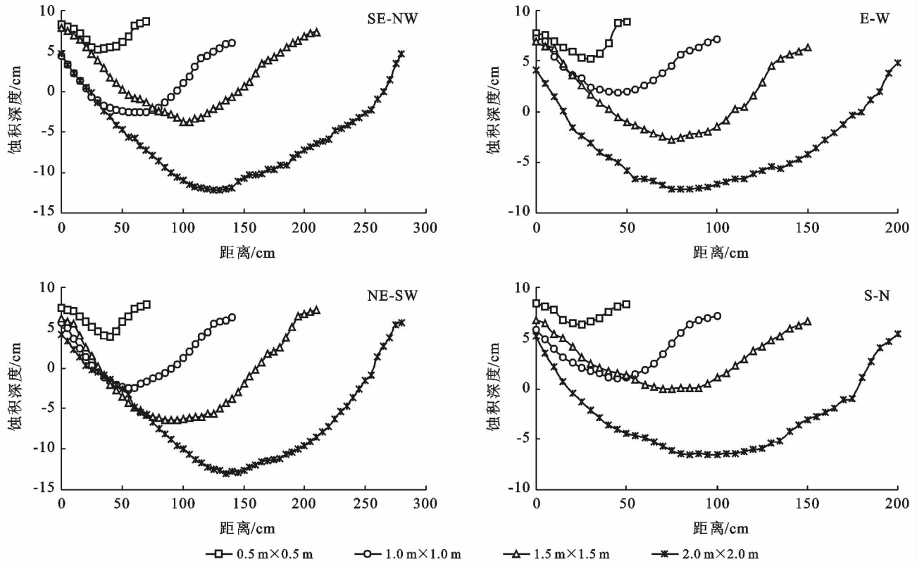
图 2 障格内不同方位蚀积深度状况
