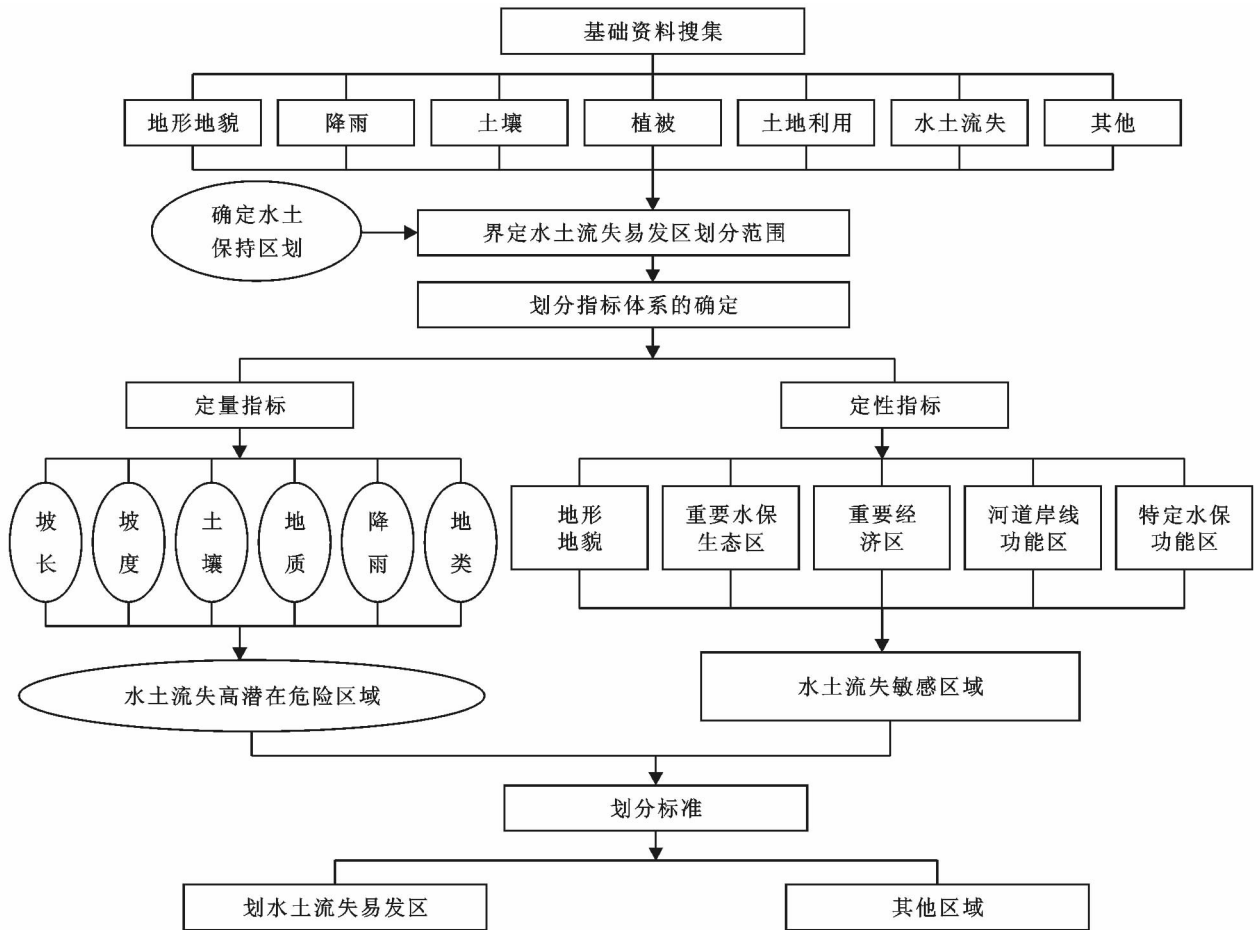
图 1 中山市平原河网区水土流失易发区界定技术路线图
