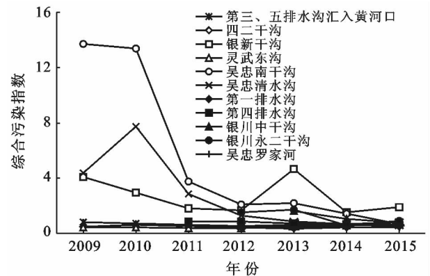
图 1 综合污染指数变化趋势
