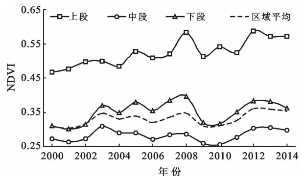
图 2 研究区各河段 NDVI 年际变化
