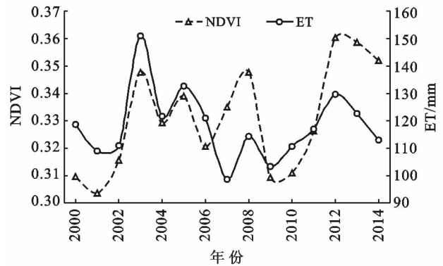
图 1 研究区全区 NDVI 和 ET 年际变化
