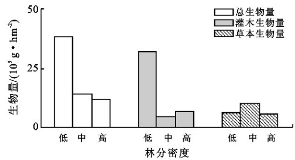
图 1 不同密度林分林下植物生物量
