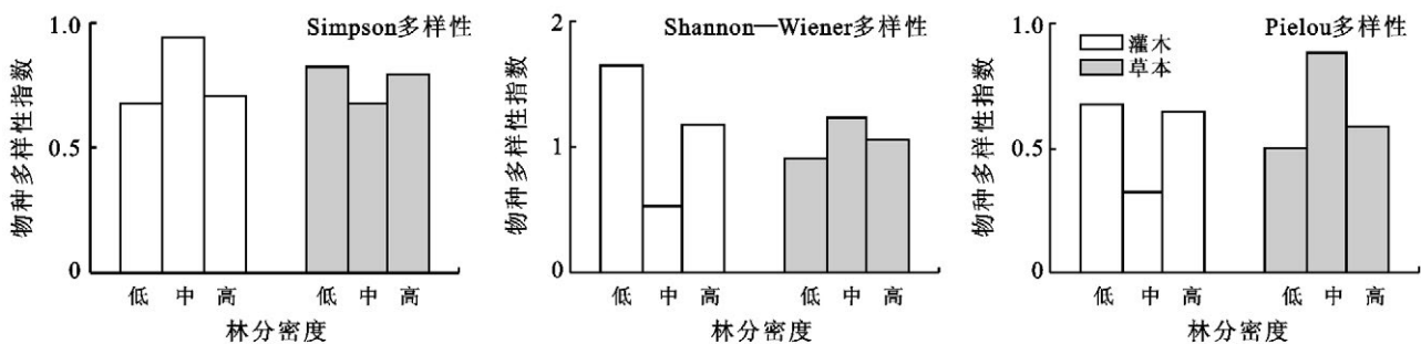
图 2 不同密度林分林下物种多样性指数
