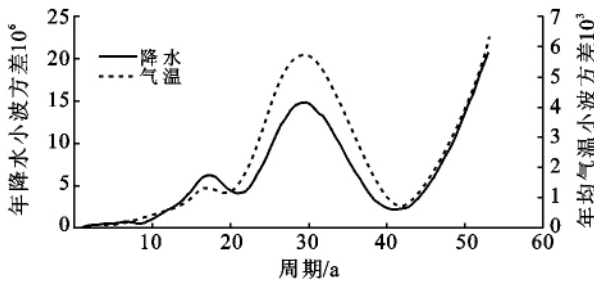
图3 渭河流域年降水量和年均温的 Morlet 小波方差
